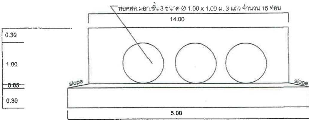
รูปด้าน - ๑ 1:100
