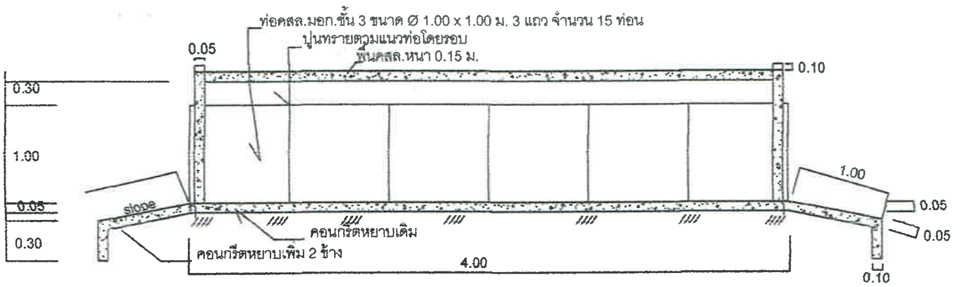
รูปตัด ๑ - ๑ 1:100
