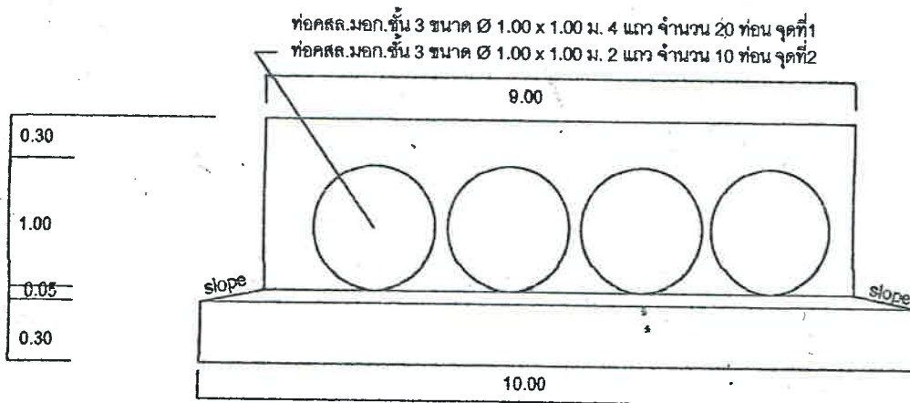
รูปด้าน - ๑ 1:100
