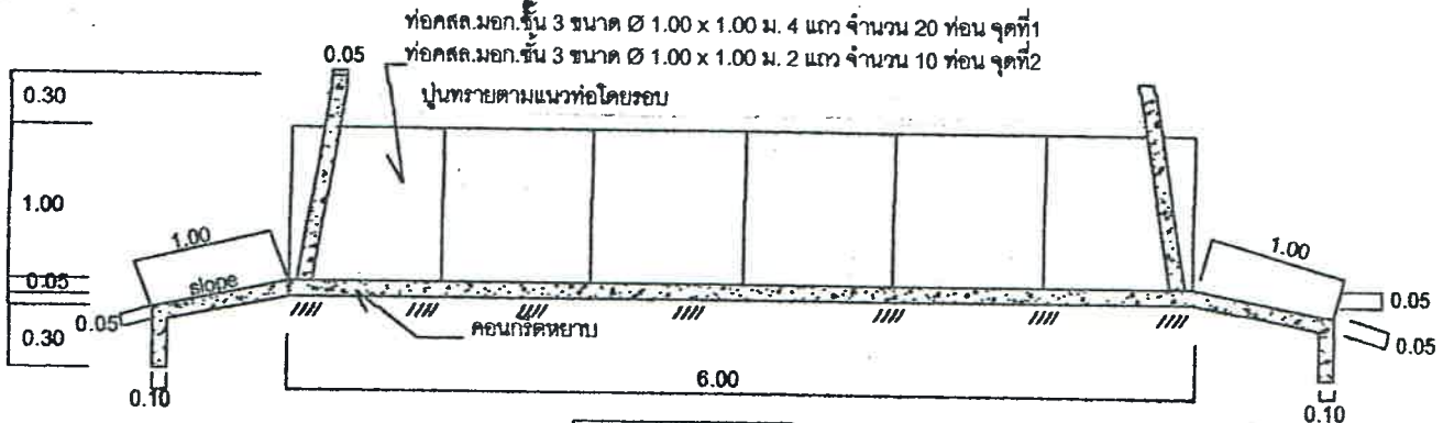
รูปตัด ๒ - ๒ 1:100
