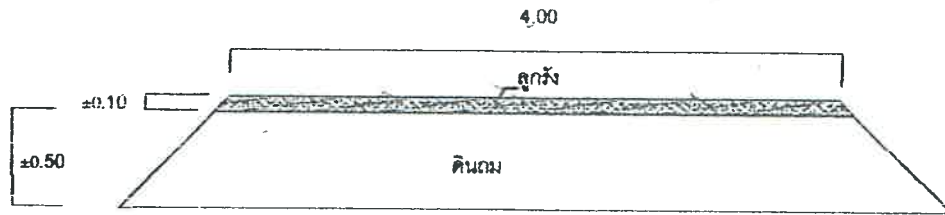
รูปตัด - 1:100
