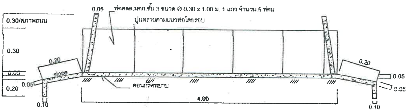
รูปตัด - 1:100
