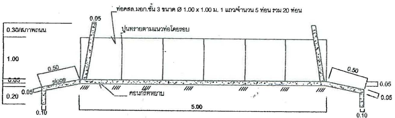
รูปตัด - ๒ - ๒ 1:100
