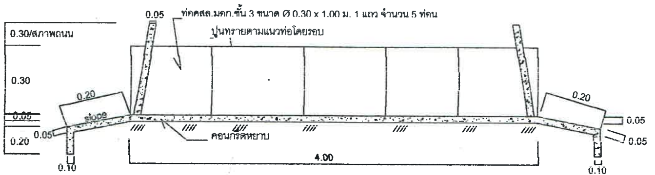
รูปตัด ๑ - ๑ 1:100
