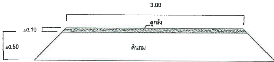
รูปตัด ๑ - ๑ 1:100
