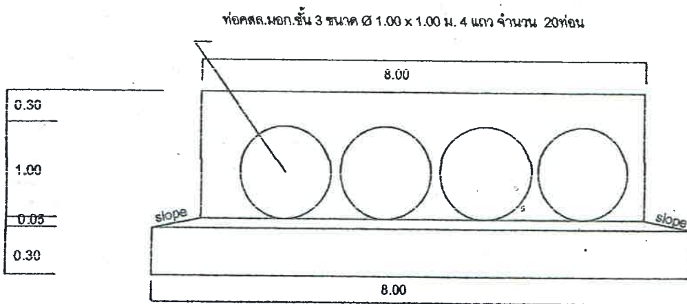
รูปด้าน - ๑ - ๑ 1:100
